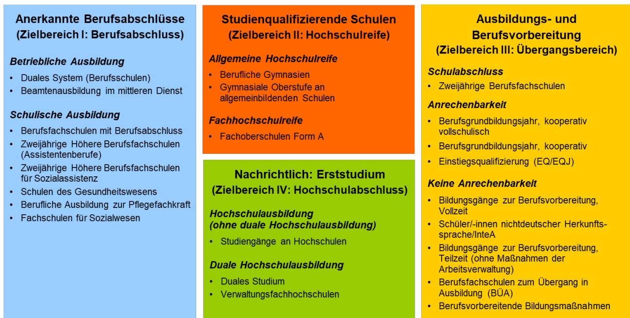
Abbildung 1: Das Zielbereiche-Modell
